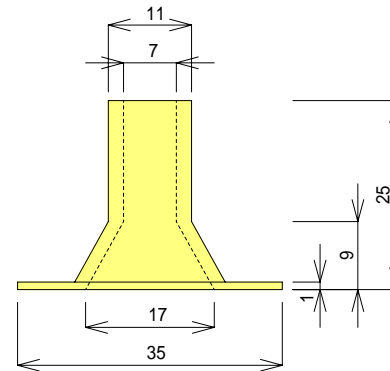
パイプ受 (大)
